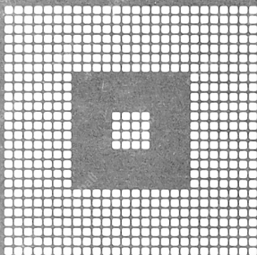
TMS320DRA342AZDK
